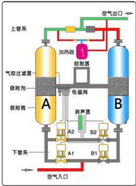
微热再生吸附式干燥机工作原理
