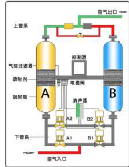
无热再生吸附式干燥机工作流程
